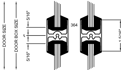
2 OPTIONAL MUNTIN DETAIL
